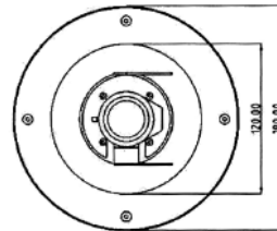
* TOP VIEW : HT-INTD3 & D4
